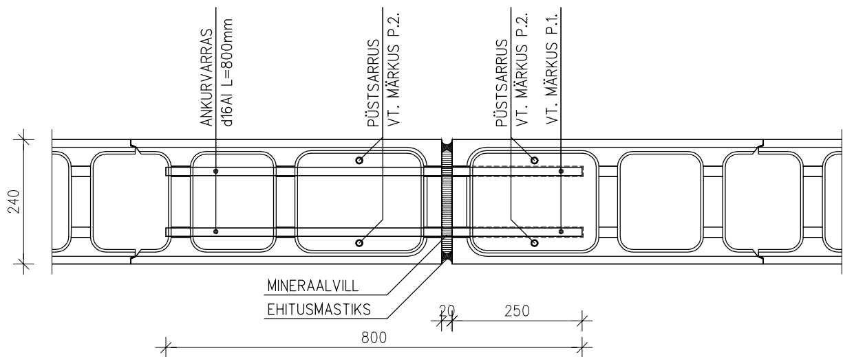
LÕIGE A-A
